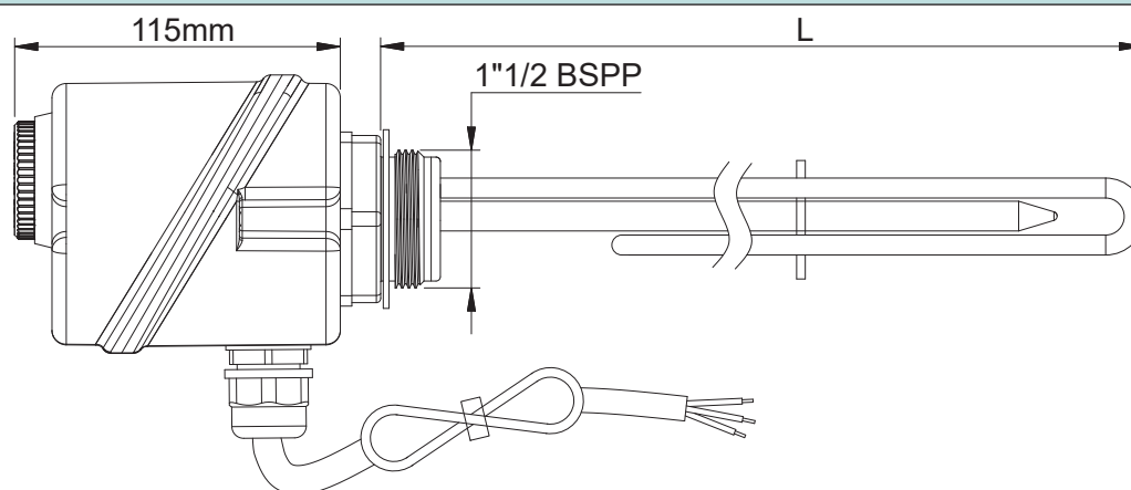
1-poliger 230V-Heizer
